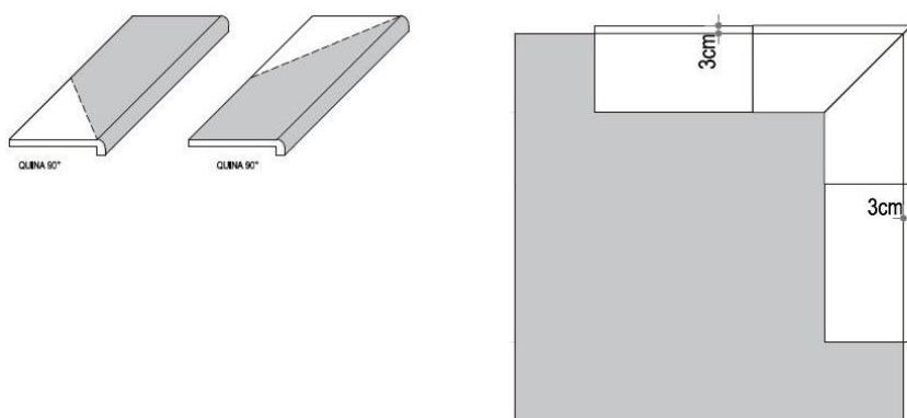
FIGURA 21. QUINA 90° FECHADA
