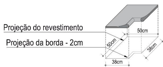
FIGURA 11. BORDA INVERTIDA
