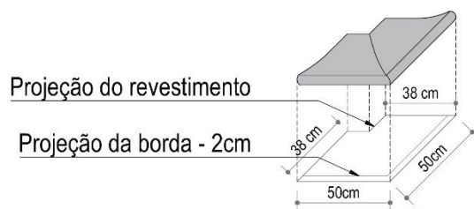
FIGURA 12. BORDA CANTO
